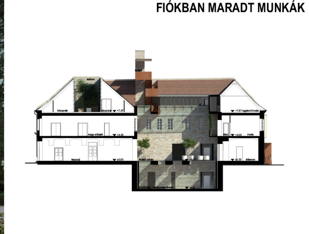
Bp. I. Úri u. 72. Műemléki épület rekonstrukciója Meghívásos tervpályázat
